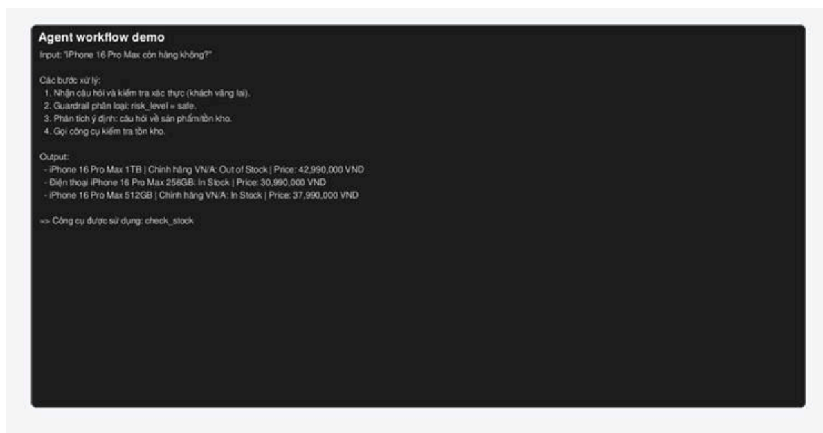
Hình 6. Agent workflow xử lý truy vấn tồn kho
